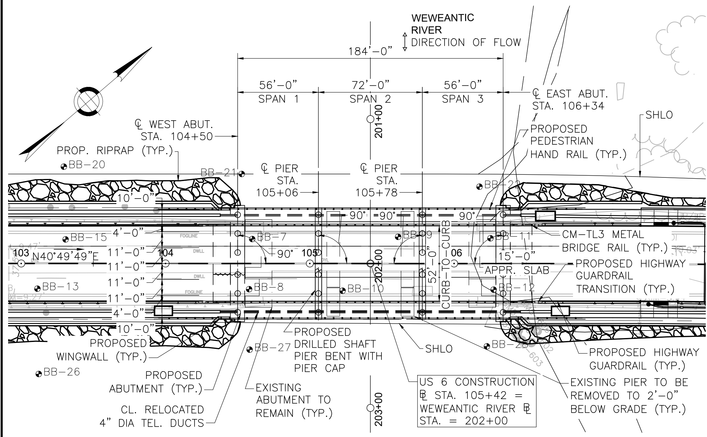
KEY PLAN SCALE: 1" = 40'
