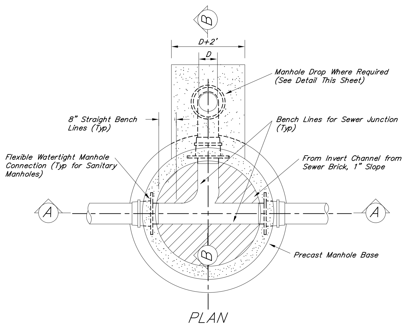
STANDARD (48") MANHOLE DETAIL Scale: 1/2"=1'-0"
