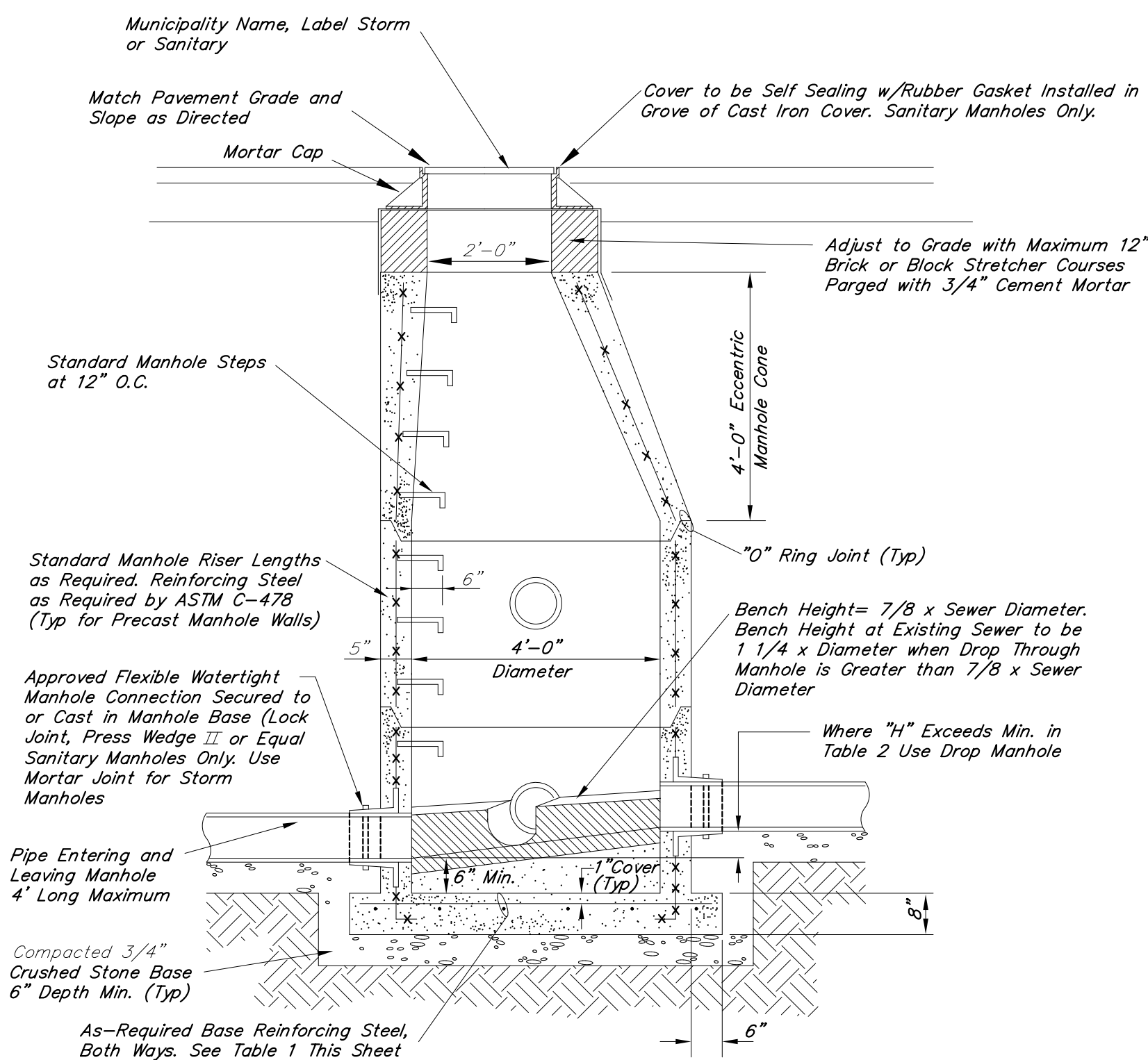
SECTION A-A
