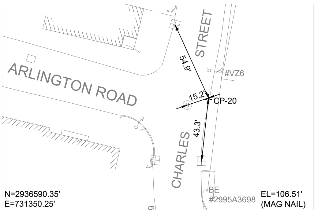
TRAVERSE SKETCH CP-20 (N.T.S.)
